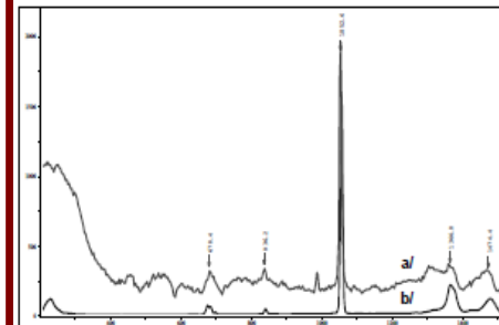
Spectre Raman d'une couche picturale (a/) comparé à celui du blanc de plomb (b/). Un des composés de cette couche correspond à de la céruse.
